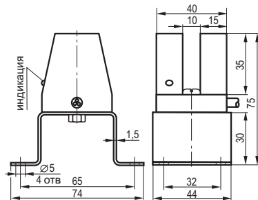
Габаритный чертёж
